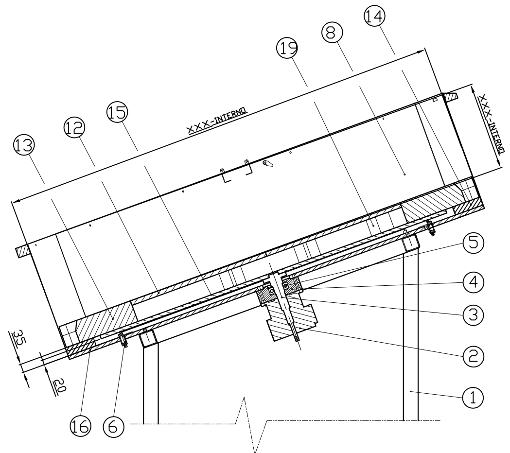
SEZIONE A-A
